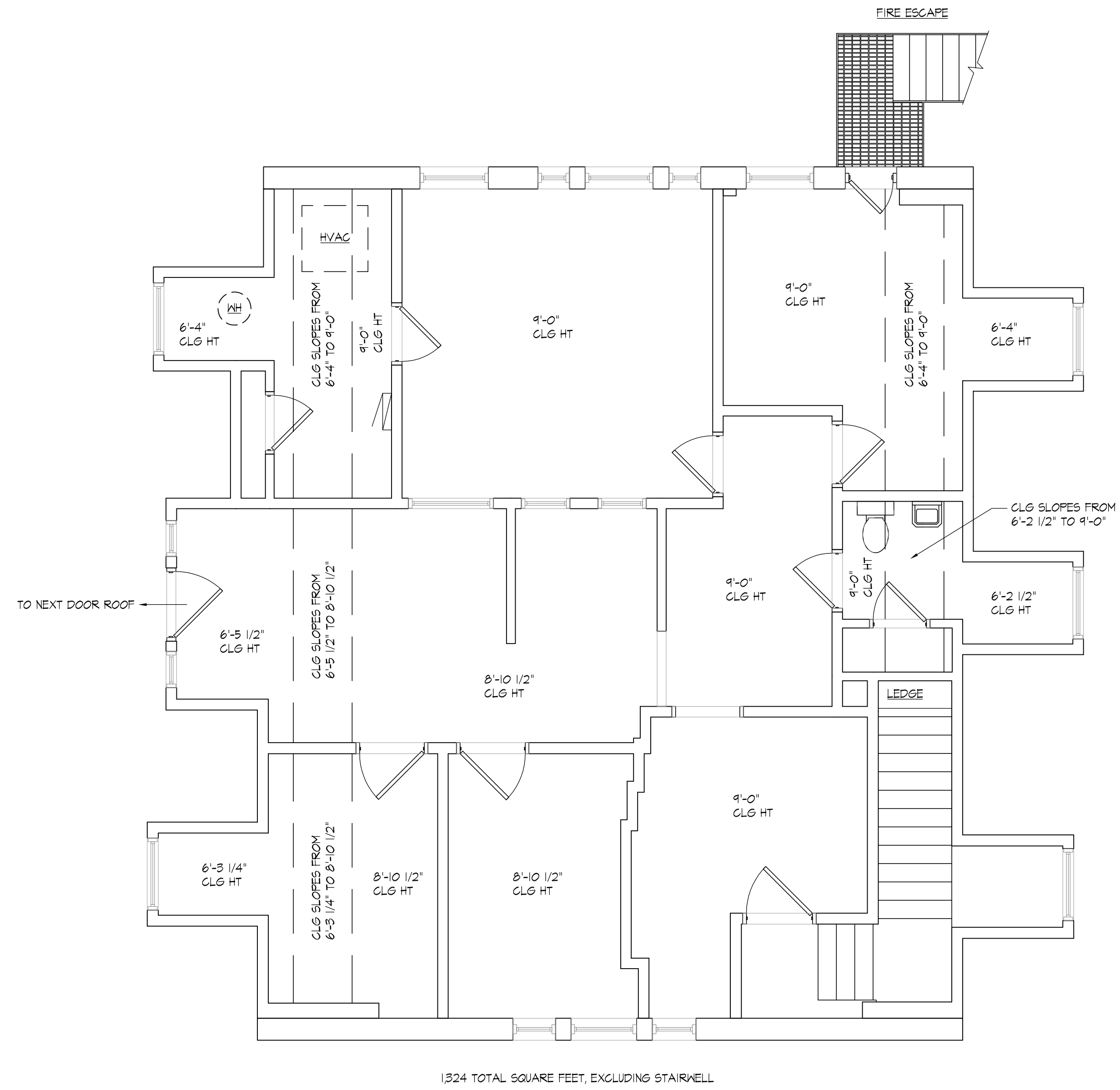
1 FLOOR PLAN A1 Scale: 1/4" = 1'-0"
